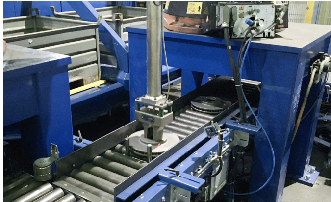
Umgebaute Verpackungszelle mit zwei Robotern, Magnetgreifern und Schwerlastdrehtisch
